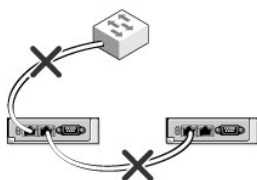
Figure 2-4. Mauvais câblage pour la connexion réseau CMC - 2 CMC
