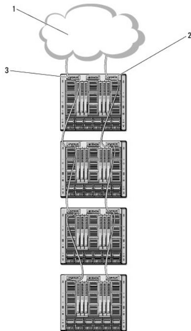
Figure 2-1. Connexion réseau CMC en chaîne
