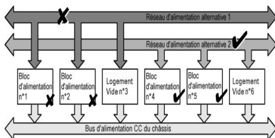
Figure 9-1. 2 unités d'alimentation par réseau et une panne électrique sur le réseau 1
