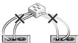
Figure 2-2. Mauvais câblage pour la connexion réseau CMC - 2 CMC
